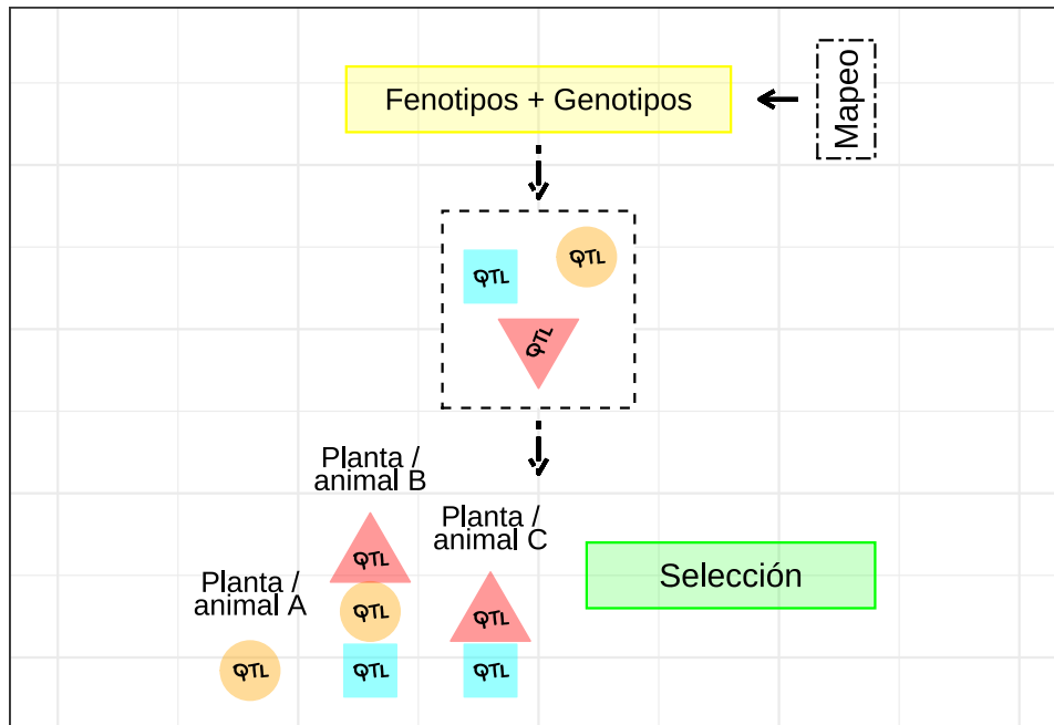
Figura 2.2: Esquema de la MAS. En la MAS, los fenotipos y genotipos de la población de mapeo se analizan usando un modelo estadístico, identificando con ello relaciones significativas entre fenotipos y genotipos. Por último, se seleccionan los individuos favorables con base en datos de genotipo. Figura adaptada de Nakaya y Isobe (2012).
