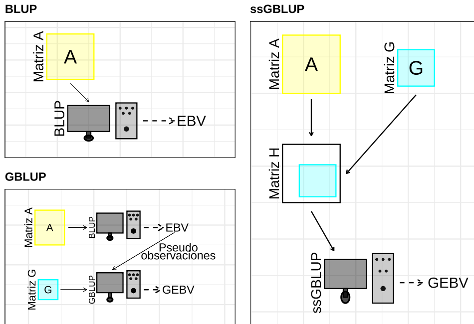
Figura 2.7: Esquema de comparación del BLUP, GBLUP y ssGBLUP. El GBLUP es un proceso de tres pasos en el que los individuos, con base en su información fenotípica y de pedigrí, son evaluados inicialmente mediante el BLUP; luego, a partir de los pseudo-fenotipos resultantes de esta evaluación inicial, se lleva a cabo un análisis genómico de los individuos genotipados mediante el GBLUP. En el ssGBLUP se simplifica este proceso al incorporar la información genómica (la matriz G) desde el primer paso.
